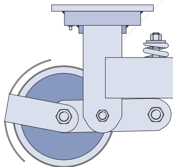
PA - Guardabarros
